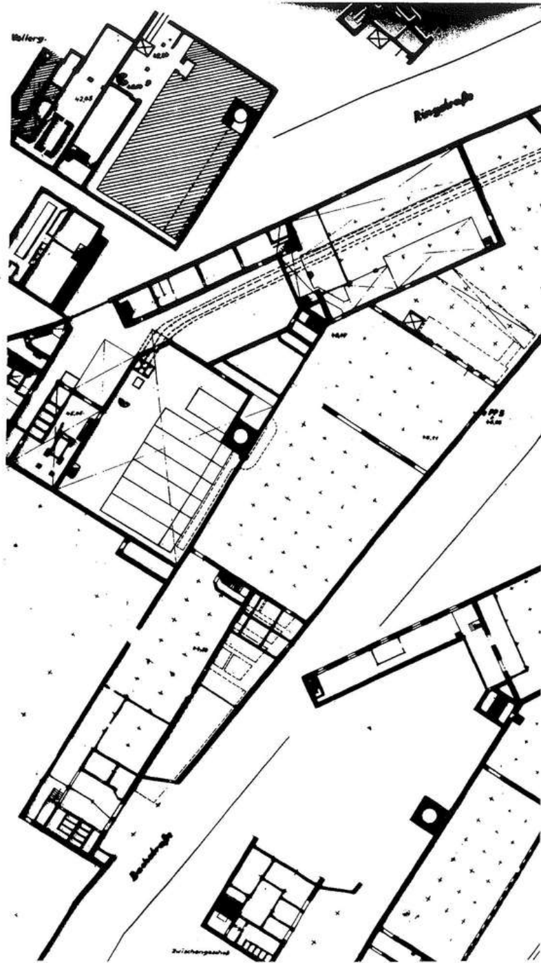
Grundriss_EG_Ringstr_Bachstr.
